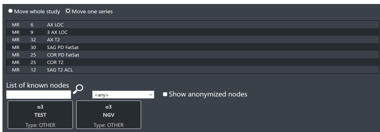
Immagine 83: Spostamento di una serie a un nodo DICOM: scelta della serie
